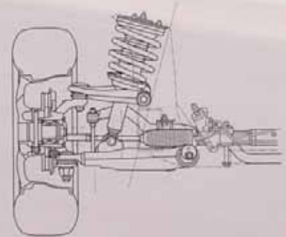
تعليق أمامي مزدوج (wishbone).
