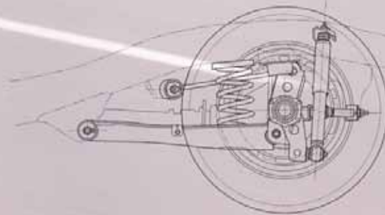
تعليق خلفي رباعي الوصلات.
